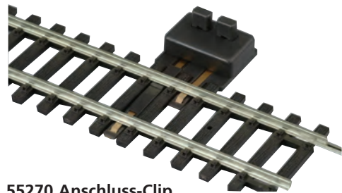
55270 Anschluss-Clip Anschluss-Clip mit EMV-Entstörelement. Passend zu G231
