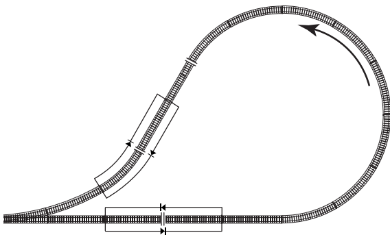
55391 Kehrschleifengarnitur Kehrschleifen-Garnitur zum problemlosen Befahren von Kehrschleifen. Bestehend aus Isolierverbindern, Kabeln und Anschlussverbindern. Nicht einsetzbar für Digital-Betrieb.
